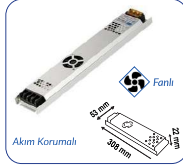
12V 25A 300W ULTRA SLİM TRAFİ
