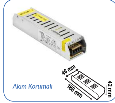
24V 8.5A 200W SLIM KASA TRAFO
