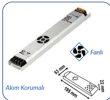
12V 16.5A 200W ULTRA SLİM TRAFİ
