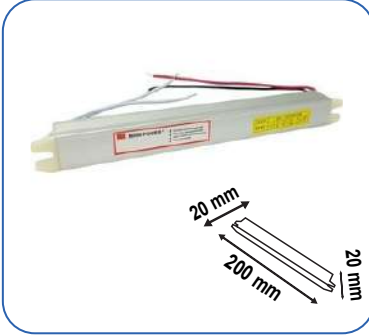
12V 3A 36W KALEM TİPİ TRAFİ
