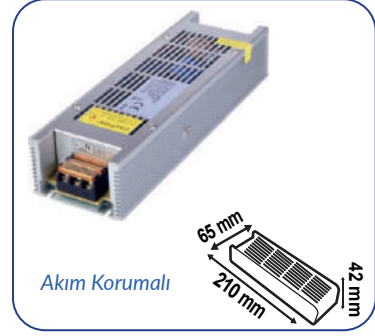
24V 20A 500W SLIM KASA TRAFO
