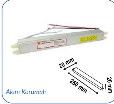
12V 5A 60W KALEM TİPİ TRAFİ
