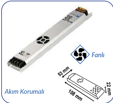
12V 5A 60W ULTRA SLİM TRAFİ
