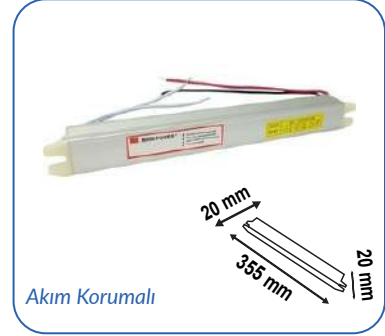
12V 6A 72W KALEM TİPİ TRAFİ
