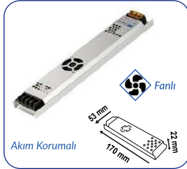
12V 10A 120W ULTRA SLİM TRAFİ
